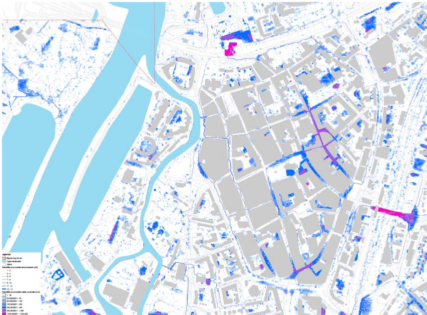
Figuur 5-1: Voorbeeld kaart met waterstromen en -diepten
