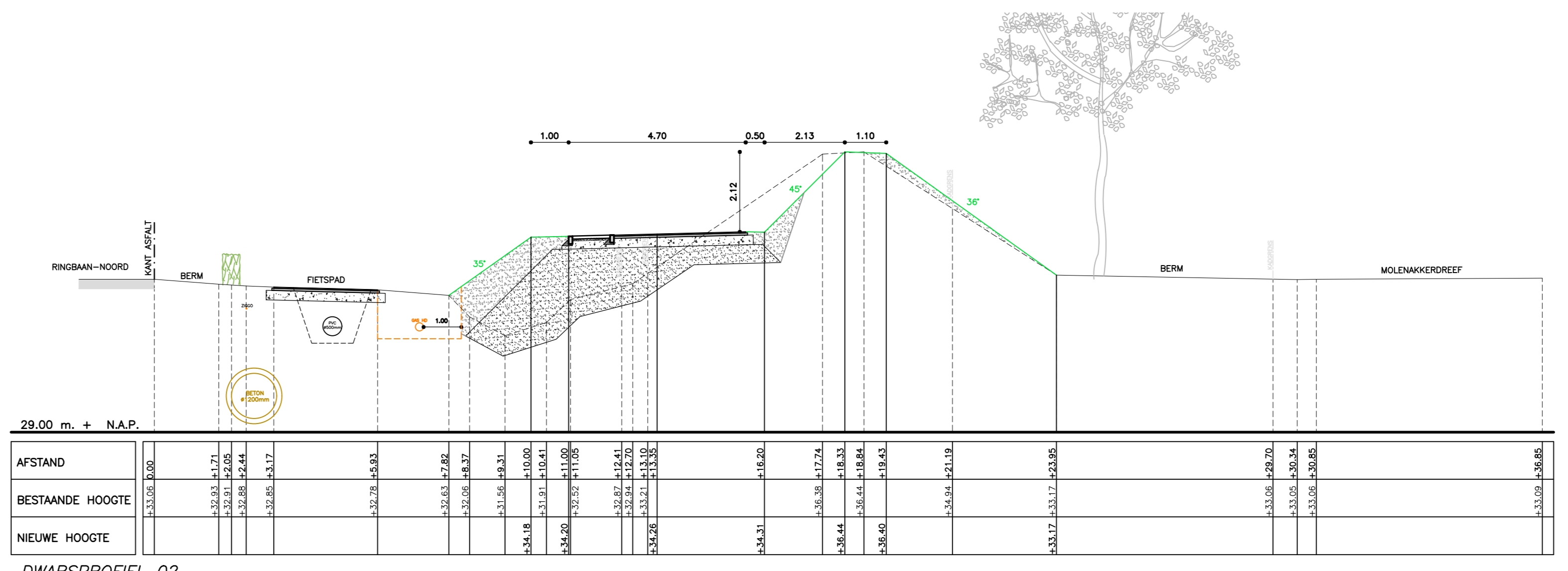
DWARSPROFIEL 02 SCHAAL 1:100
