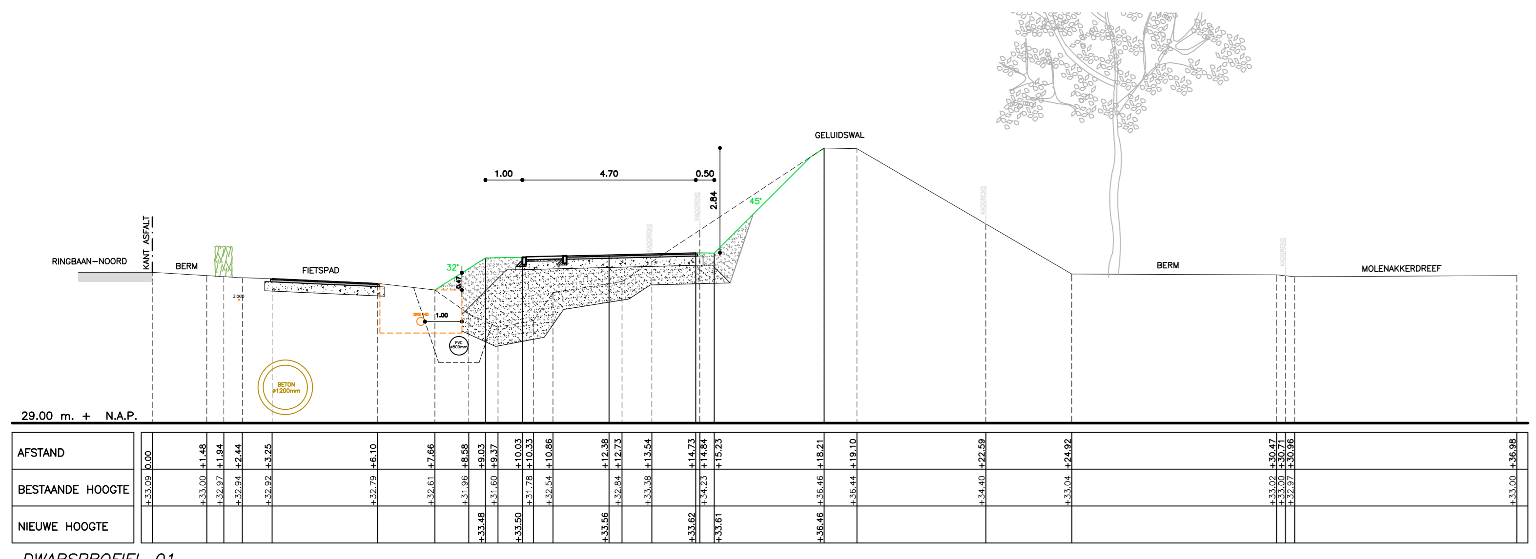
DWARSPROFIEL 01 SCHAAL 1:100
