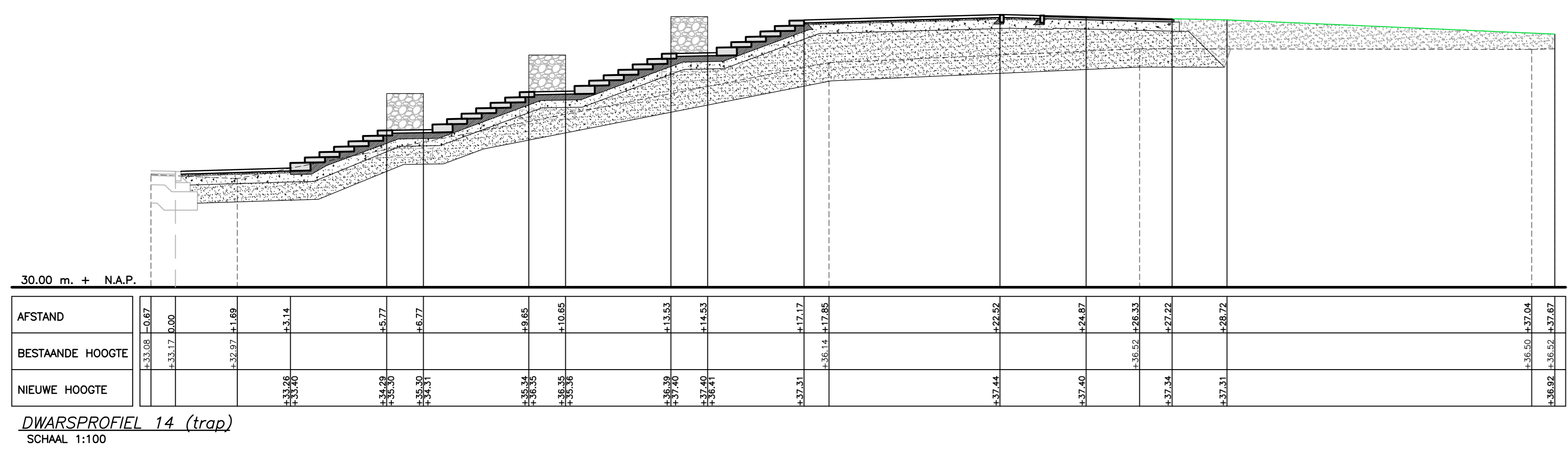
DWARSPROFIEL 14 (trap) SCHAAL 1:100
