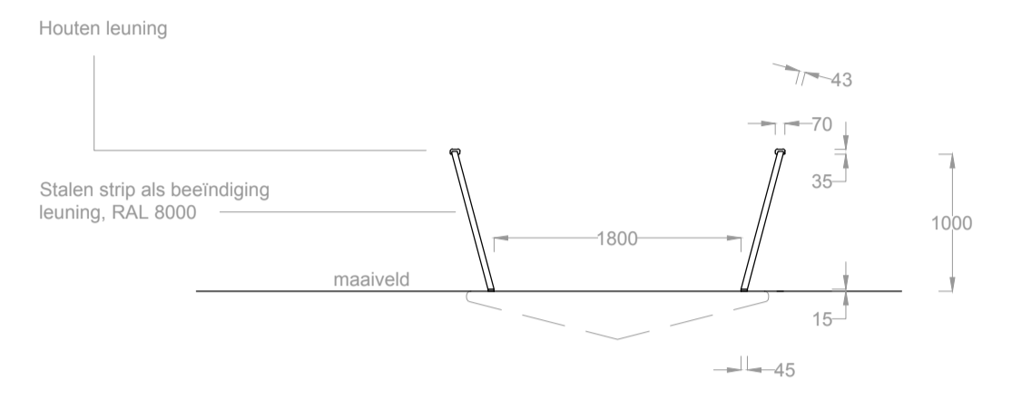
Aanzicht uiteinde brug en beëindiging leuning
