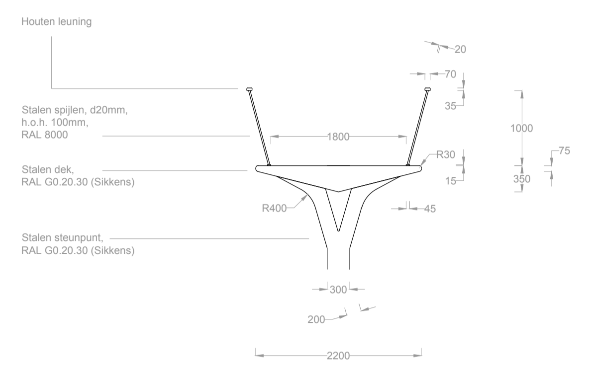
Doorsnede profiel brug met steunpunt
