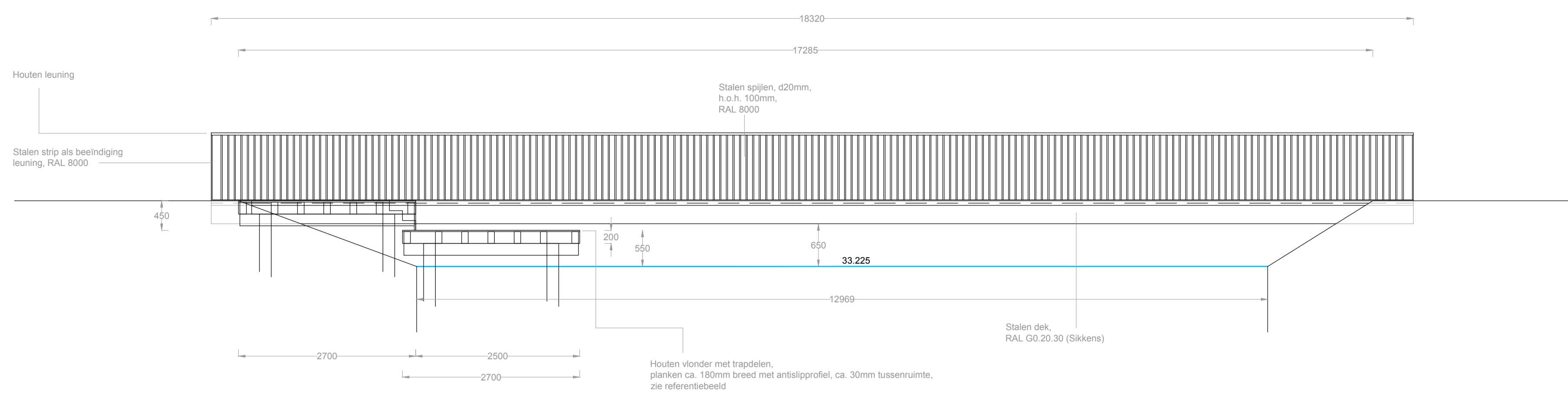
Zij-aanzicht brug en aansluiting vlinder
