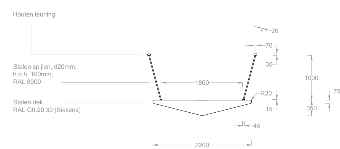
Doorsnede profiel brug, geen steunpunt
