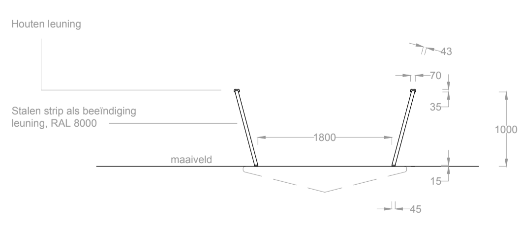
Aanzicht uiteinde brug en beëindiging leuning
