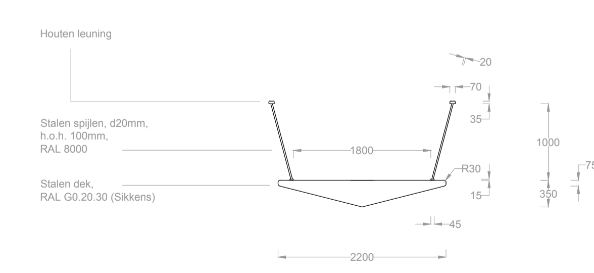
Doorsnede profiel brug, geen steunpunt
