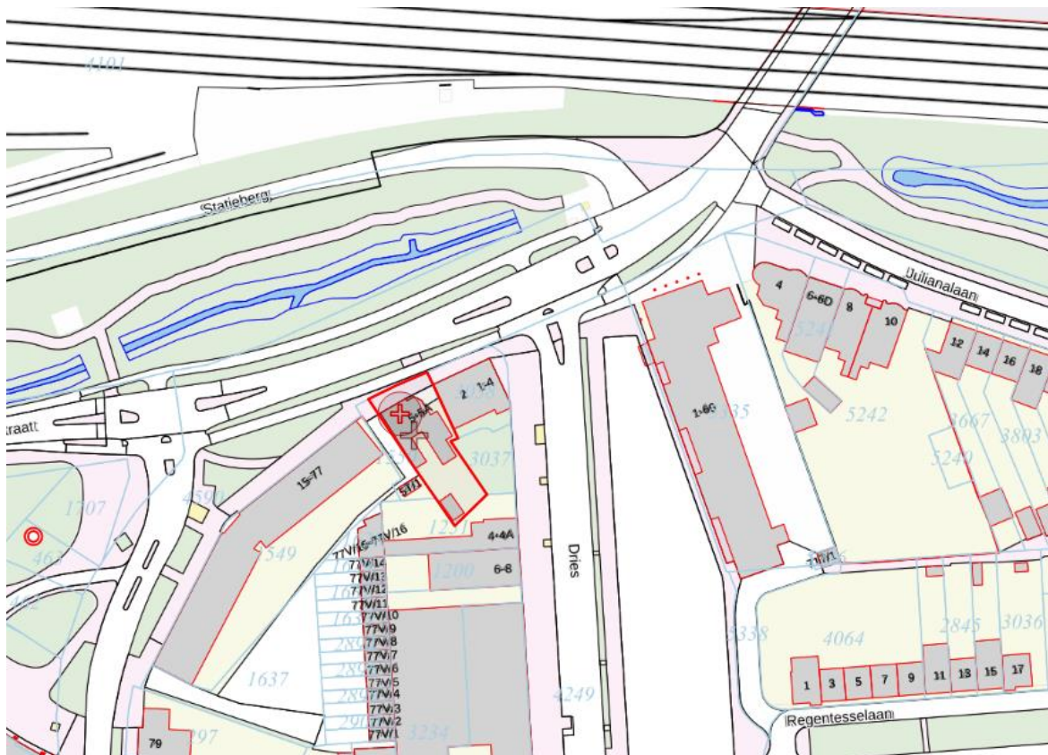
Kadastrale situatie
