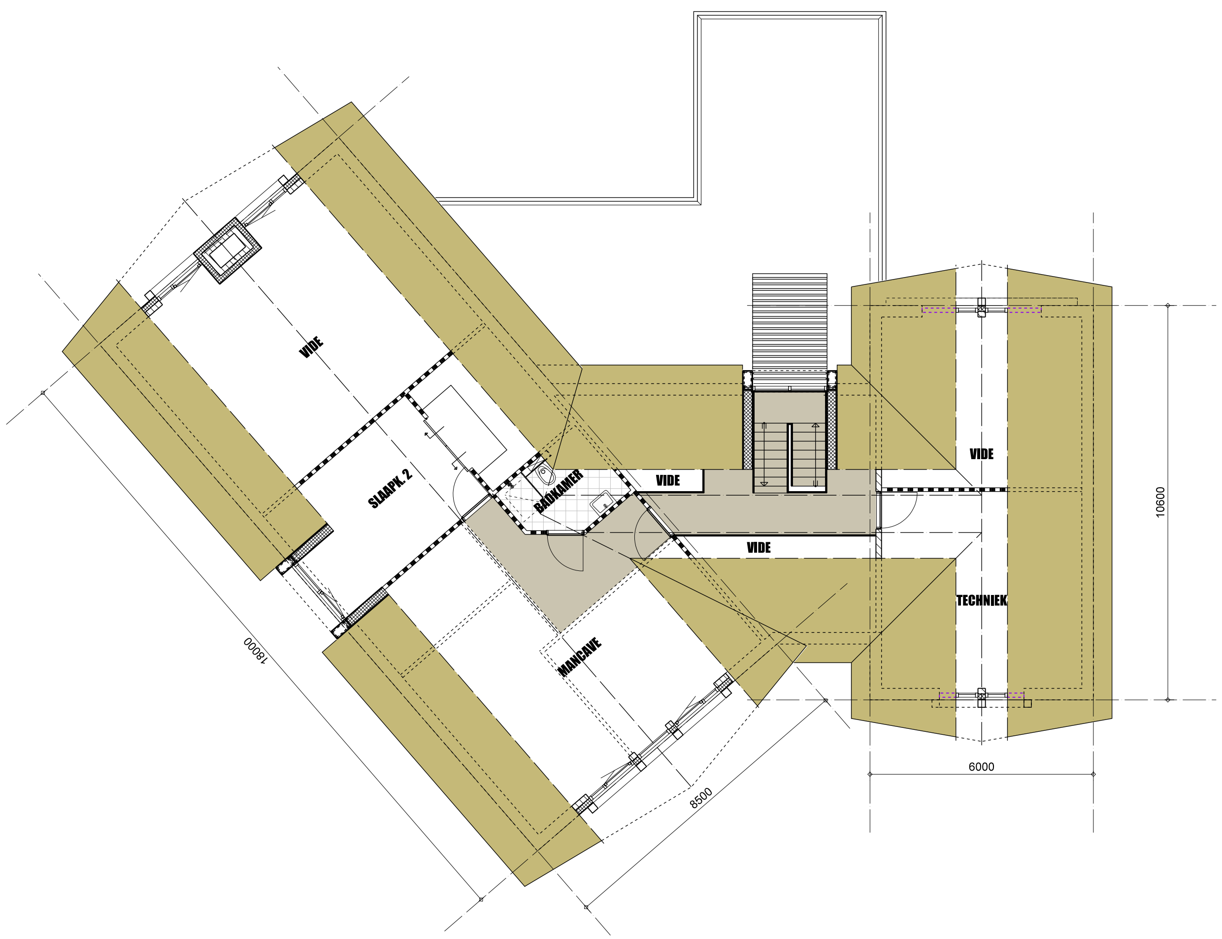
VERDIEPING
