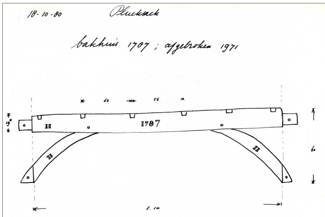
Fig. 13. Eiken ankerbalk met korbelen en telmerken, gedateerd 1787. Afkomstig uit bakhuys ten zuiden van 'De Plucksackhof'. Tekening: Alfons Bruekers.
