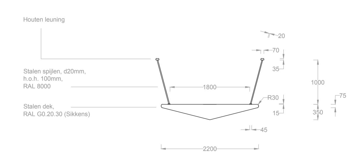
Doorsnede profiel brug, geen steunpunt
