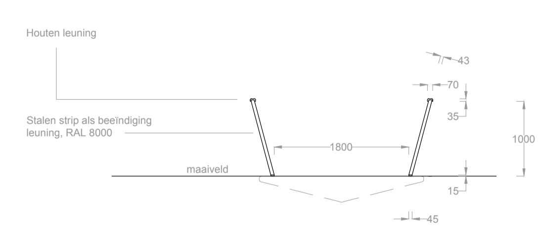
Aanzicht uiteinde brug en beëindiging leuning
