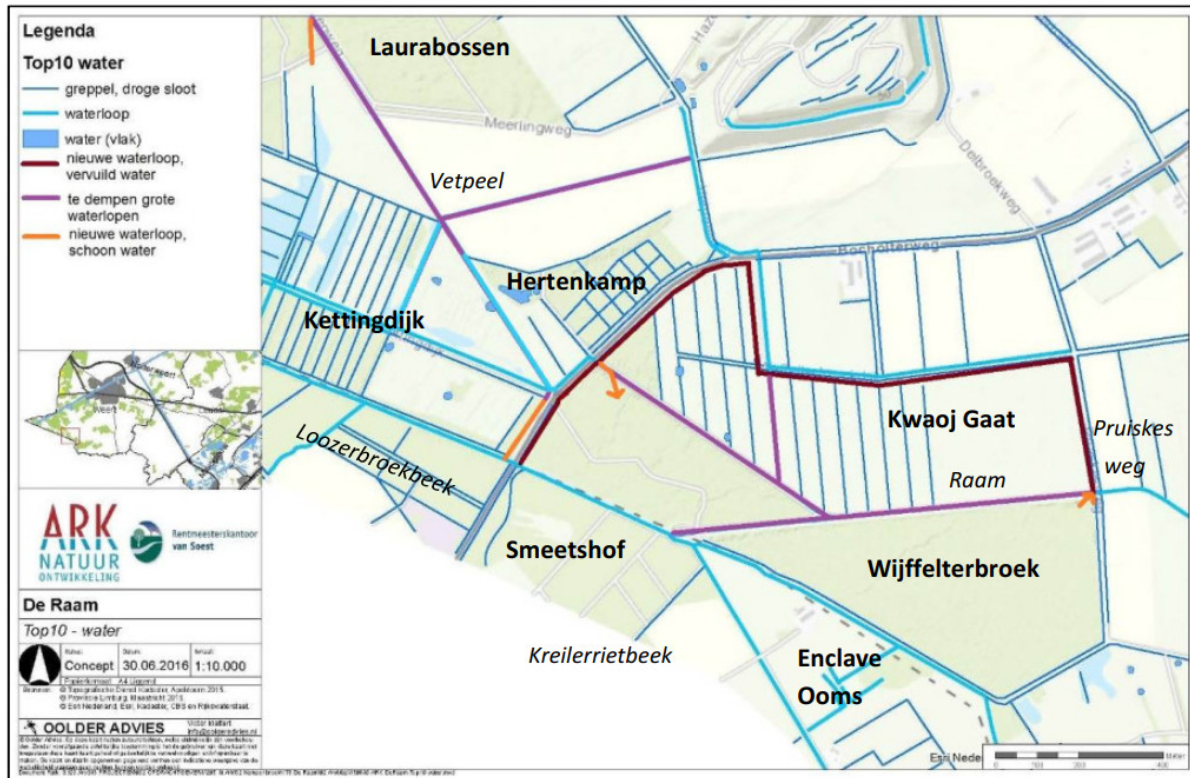
Figuur 1, Ontwerp herinrichting Wifffelterbroek en Vetpeel.
