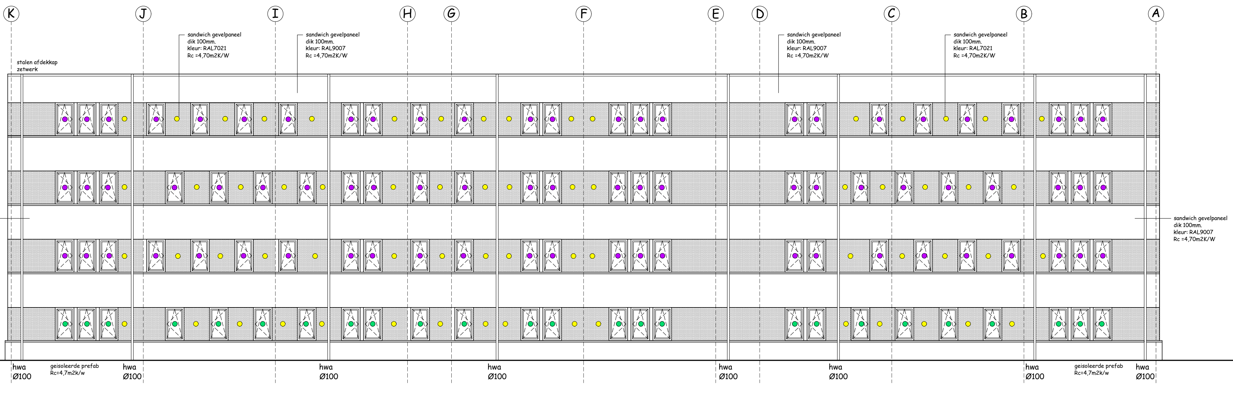
achtergevel
