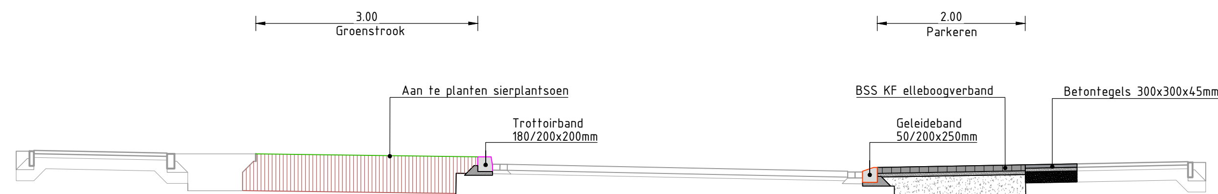
Dwarsprofiel A-A Johanna van Polanenstraat variant 2 schaal 1:50
