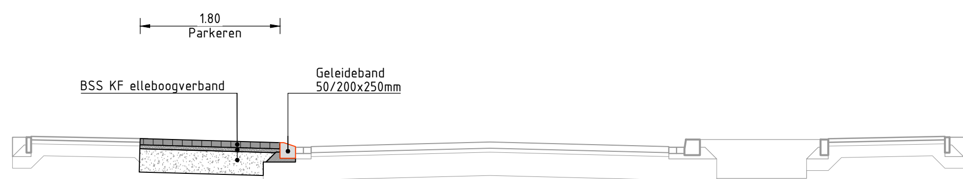
Dwarsprofiel D-D Irenelaan schaal 1:50
