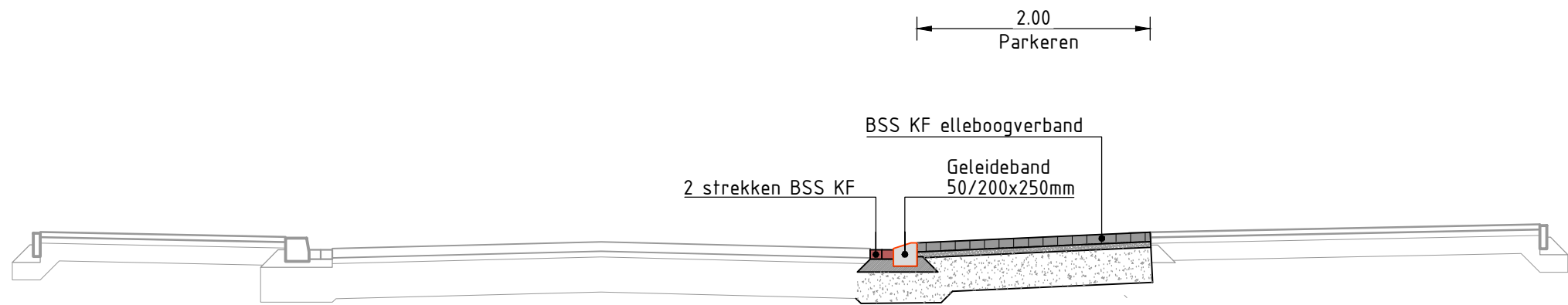
Dwarsprofiel B-B Margrietlaan variant 2 schaal 1:50
