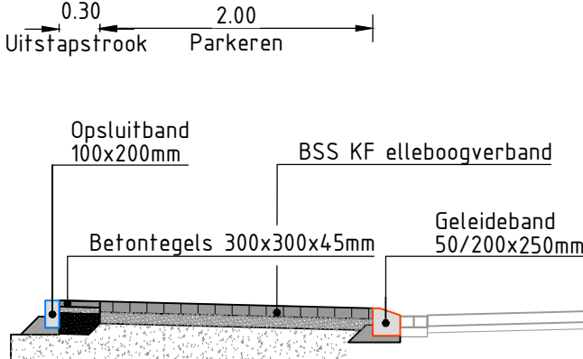
Dwarsprofiel C-C Jan de Oudestraat variant 2 schaal 1:50
