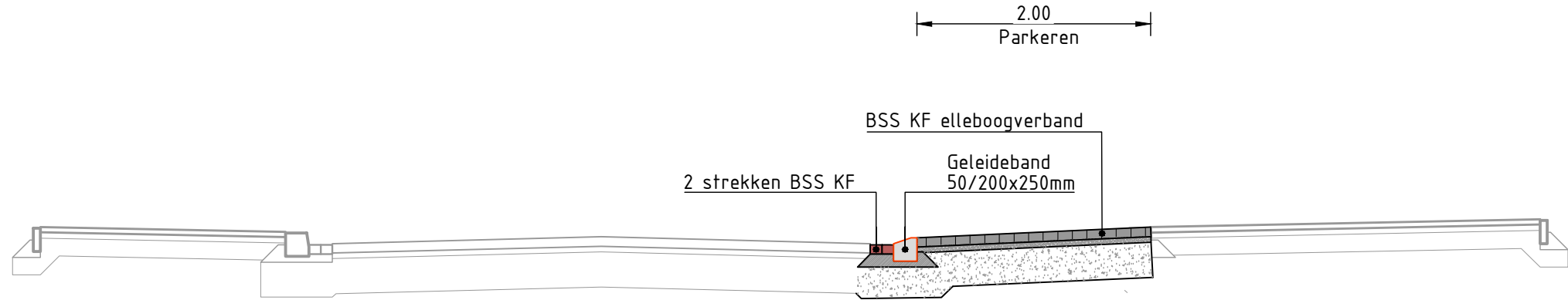
Dwarsprofiel B-B Margrietlaan variant 3 schaal 1:50
