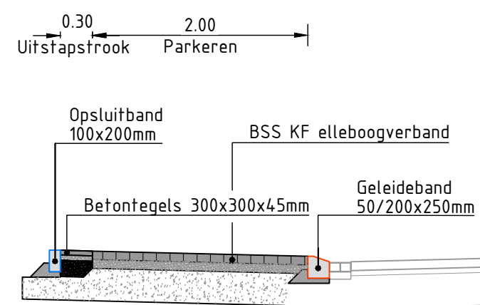
Dwarsprofiel C-C Jan de Oudestraat variant 3 schaal 1:50
