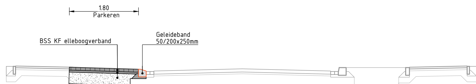
Dwarsprofiel D-D Irenelaan schaal 1:50
